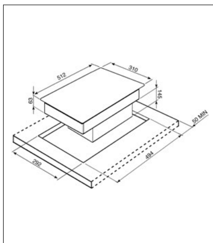
30CM DEEP-FRY HOB: PGF30F
