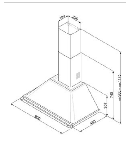
90CM EXTRACTOR: KT90PE/XE/BLE
