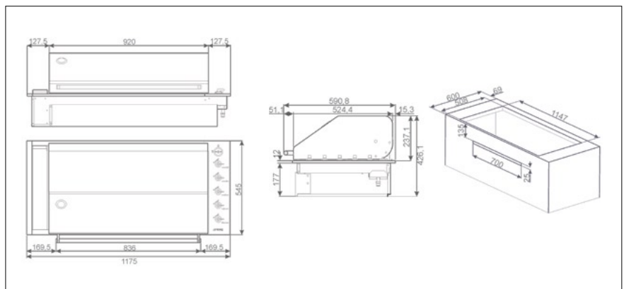
110cm GAS BRAAI: BIBQ1205H
