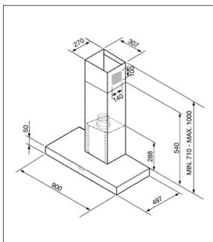
90CM EXTRACTOR: KS905SXE/BXE
