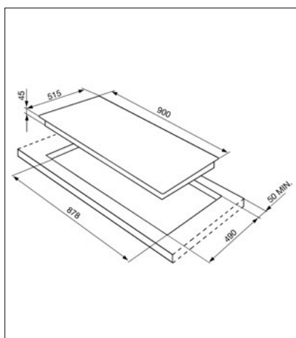
90CM INDUCTION HOB: SI5952B
