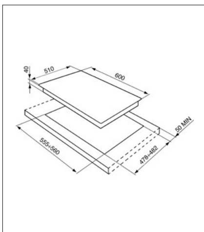
60CM & 70CM HOBS: P361XGHL; P372XGHL
