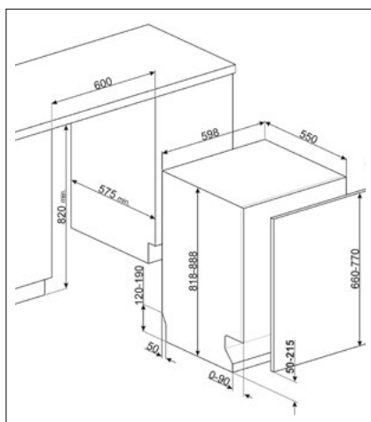
60CM DISHWASHER: DWI9QDLSA
