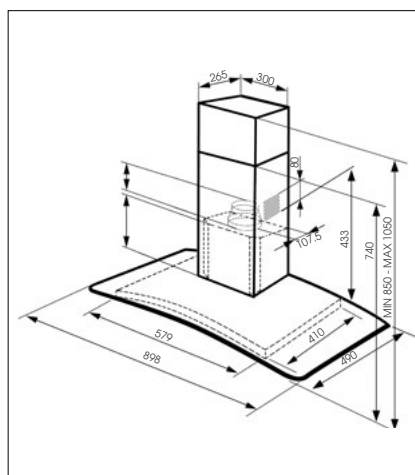
90CM EXTRACTOR: KV90XE
