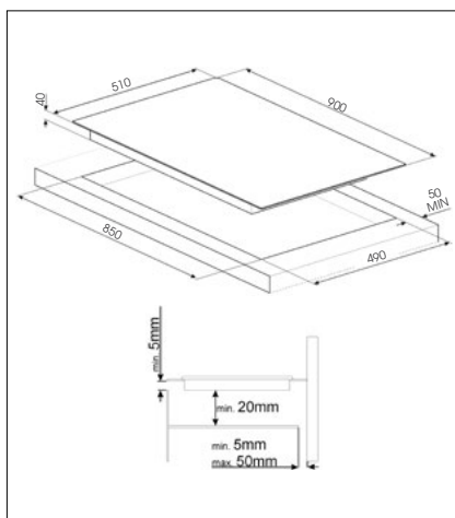
90CM CERAMIC HOB: SE395ETB
